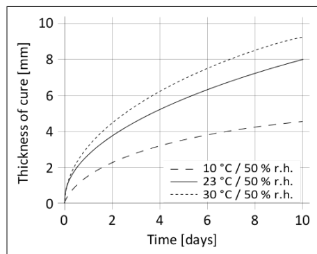
Diagrama 1: Veocidade de cura do Sikaflex®-591
